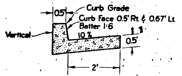
Type "B" Curb Scale: 1"=1'
