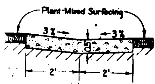
Valley Gutter Scale: 1"=1'
